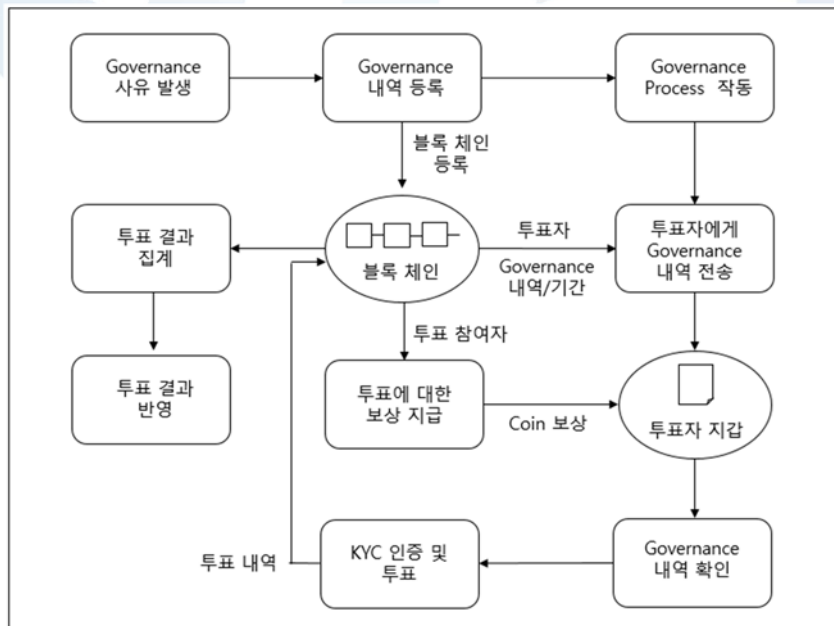
[Fig 4] Governance 개요도
